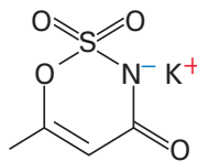
Estructura química del acesulfame K.
